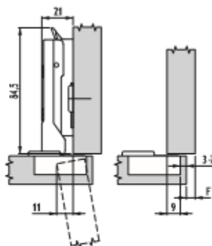
Montageplaathoogte 3
