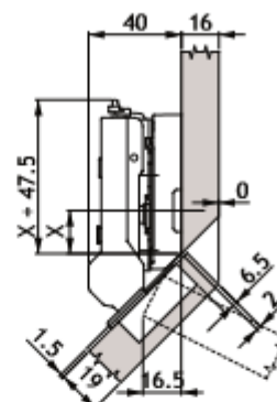
Montageplaat hoogte 12
