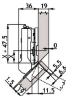
Montageplaat hoogte 8
