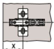
Kruismontageplaten met bevestigingsafstand 37
