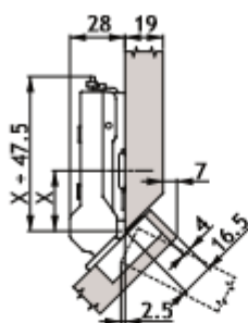
Montageplaat hoogte 0
